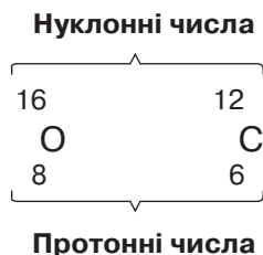
Рис. 11. Символьне позначення ядер атомів Оксигену й Карбону
